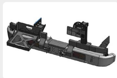
Parachoques trasero con doble soporte para rueda y bidón. 189.6153
