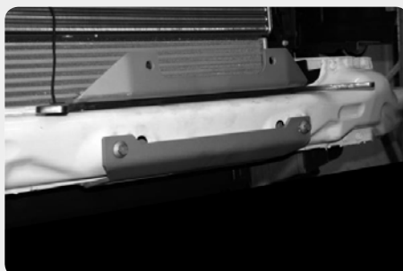
Base de cabestrante "oculta" para instalar en parachoques de origen. 189.4603
