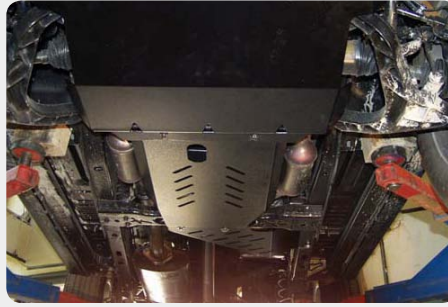
Protector de caja de cambios y caja de cambios SHERIFF. 190.04.0975 - acero zincado
